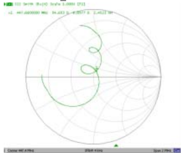
Smith Chart_S22 :
